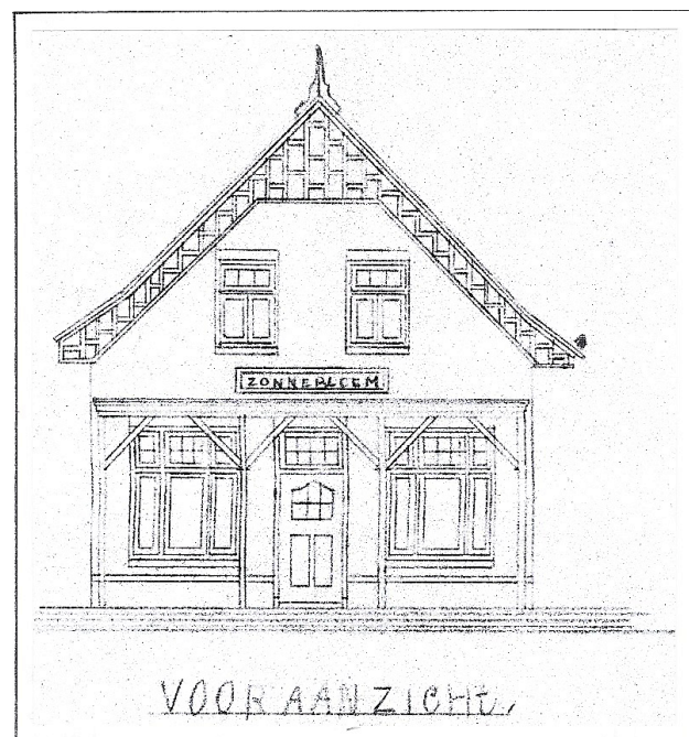
Bouwtekening van café 'de Zonnebloem' bij aanvraag vergunning voor de aanbouw van een waranda in 1939.
