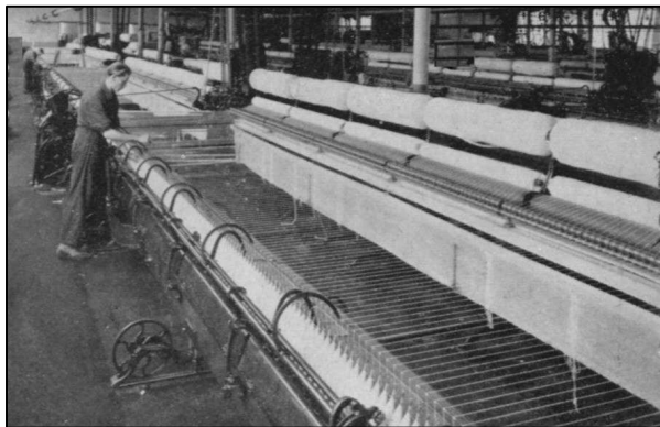
Het opspoelen der garens
