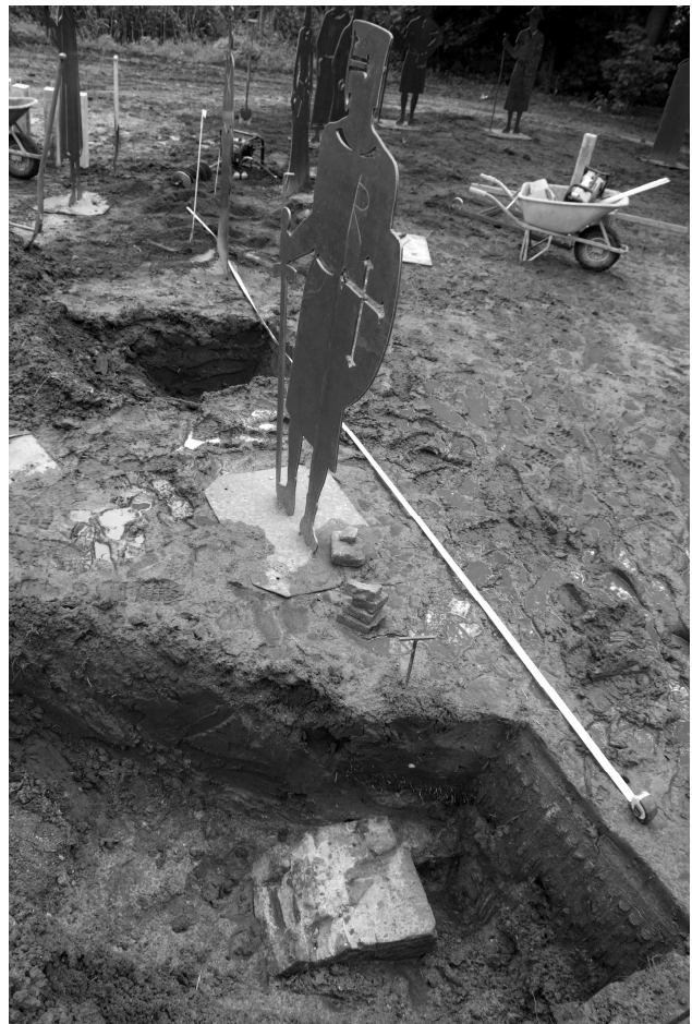
Overzichtsfoto. Op voorgrond in de kuil de eerste poer, in kuil achter kruisridder de tweede.
