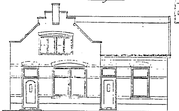
Gewijzigde voorgevel. Schaal 1:100.
